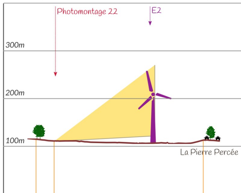
Coupe topographique (Profil Tool d'après IGN BD ALTI 25, Occupation du sol d'après Géoportail, DREAL/DRAC CVdL&IdF)
